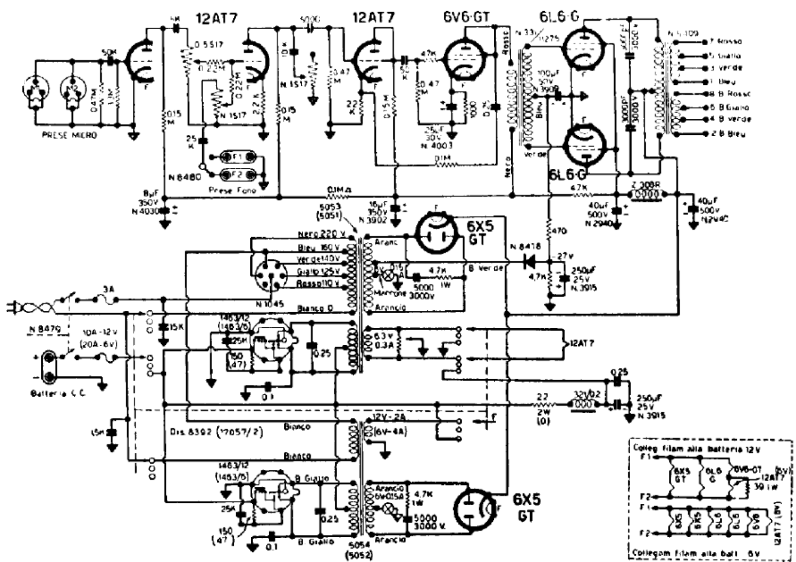
AMPLIFICATORE G. 229/12 (229/6) (S.A. S.E.L. 819 - Roma)
